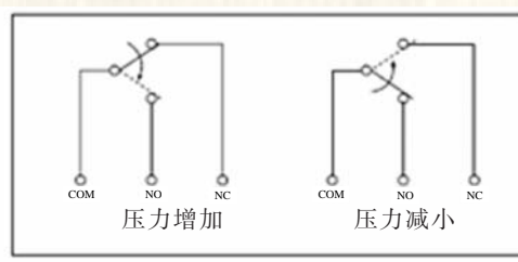
PS40A SPDT 接点动作情况
